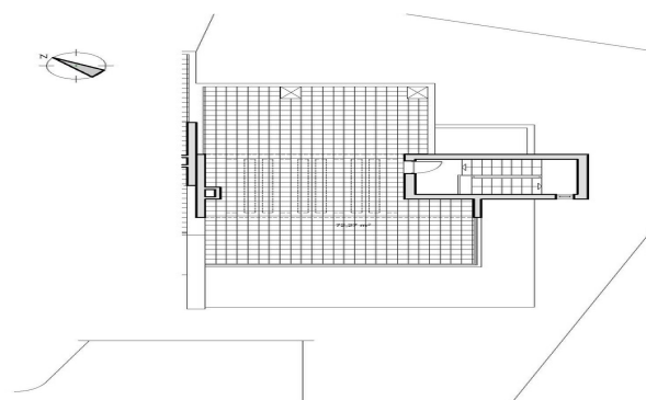
PLANTA DA AÇOTEIA - ESC. 1/100
