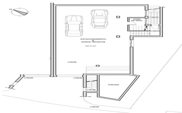
PLANTA DA CAVE - ESC. 1/100
