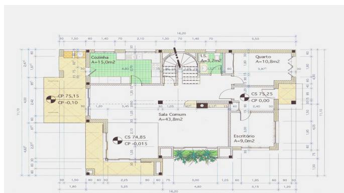
PISO 0.0 A=120,0m 2
