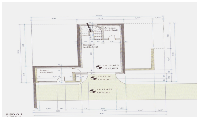
PISO 0.1 A=60,0m 2
